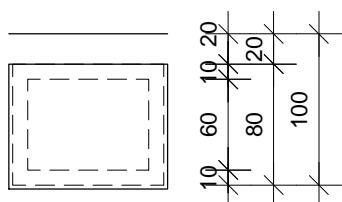
TLOCRT
