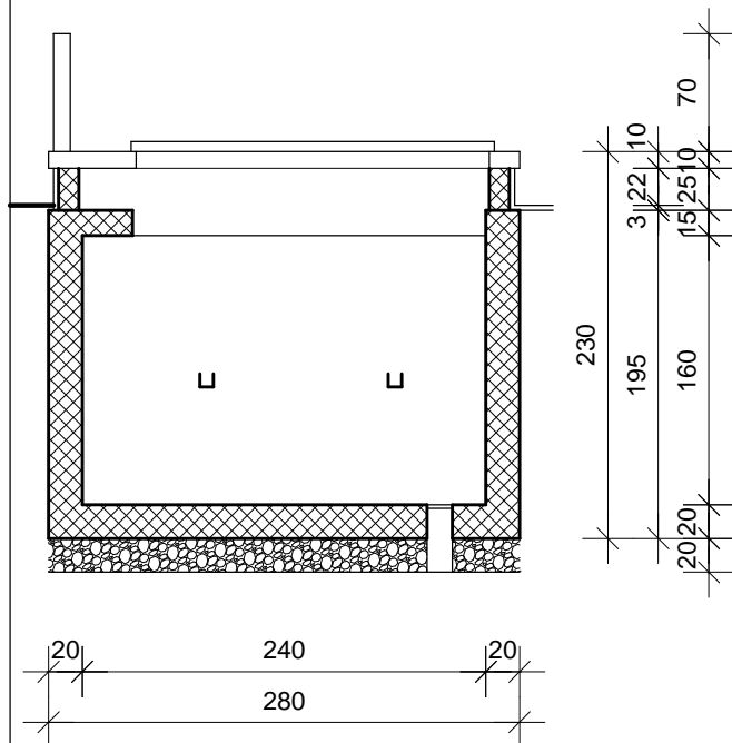
PRESJEK A-A
