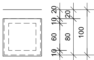
TLOCRT
