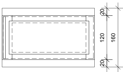
TLOCRT
