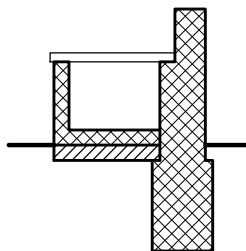
PRESJEK B-B
