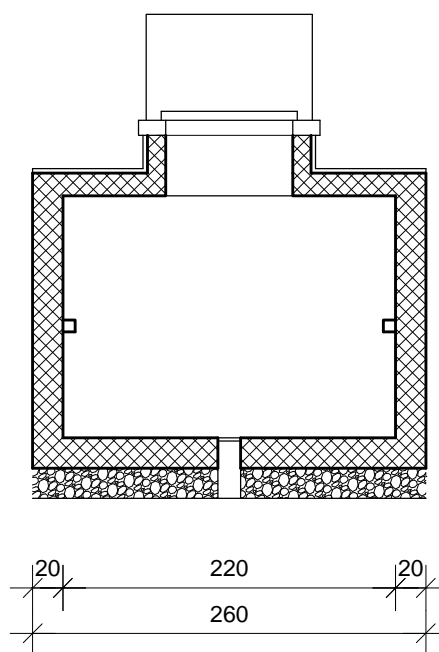
PRESJEK B-B
