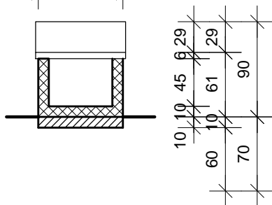
PRESJEK A-A
