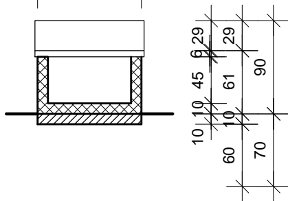
PRESJEK A-A
