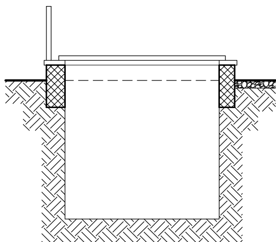
PRESJEK A-A
