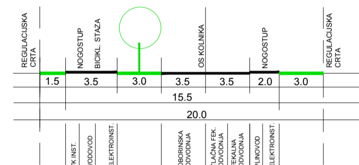
ULICA "D" _ PRESJEK 1-1
