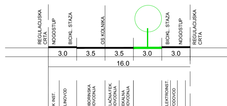
ULICA "E" _ PRESJEK 1-1
