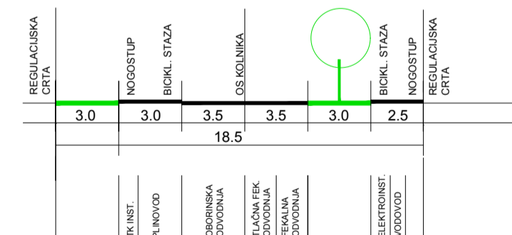
ULICA "F" _ PRESJEK 1-1
