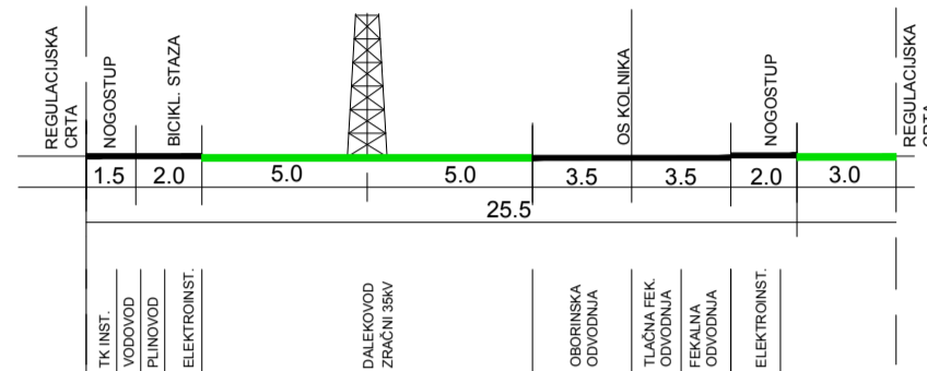
ULICA "C" _ PRESJEK 1-1_ ETAPA 2
