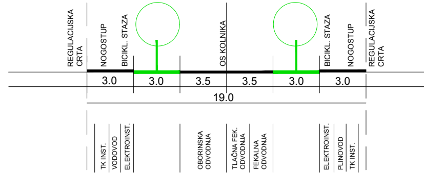
ULICA "C" _ PRESJEK 1-1_ ETAPA 1
