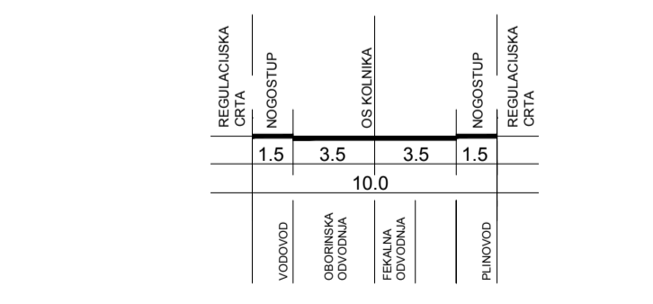
ULICA "G" _ PRESJEK 1-1
