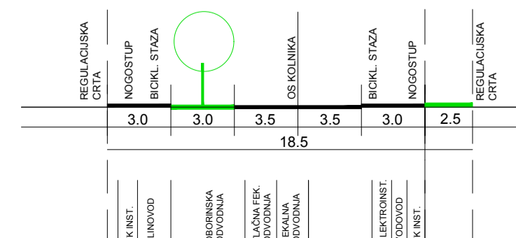
ULICA "G" _ PRESJEK 1-1
