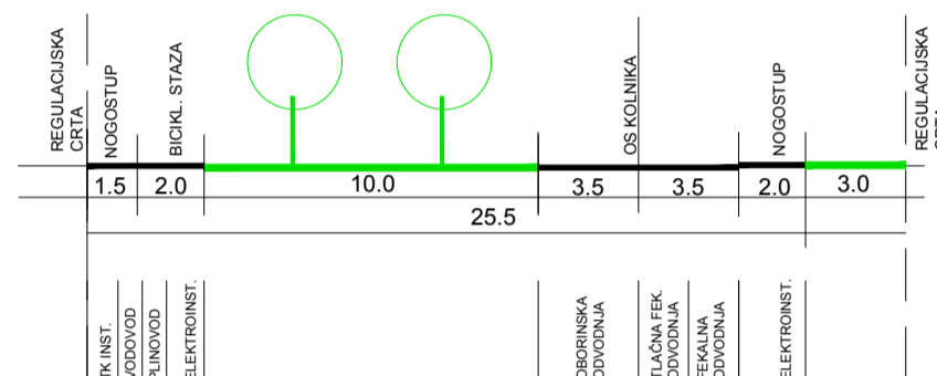
ULICA "C" _ PRESJEK 2-2
